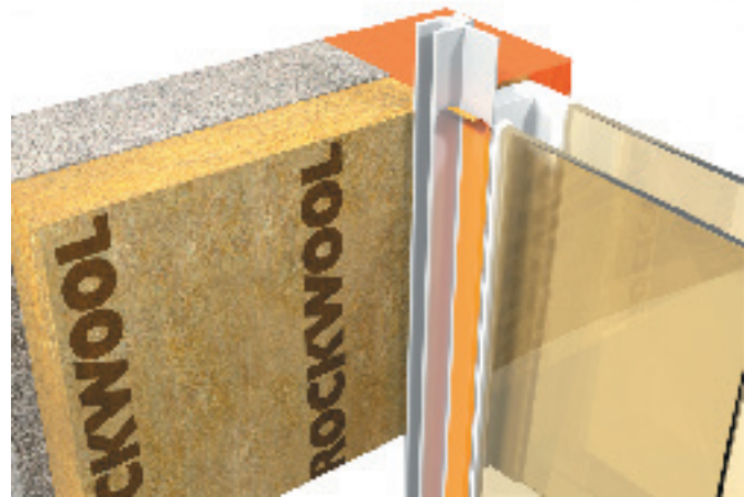
Рисунок 6. Профиль примыкающий самоклеящийся (без сетки)
